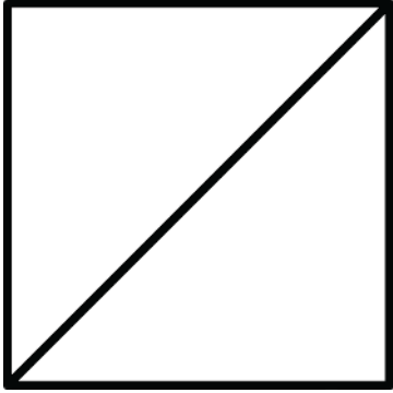
Color \frac{1}{2}
