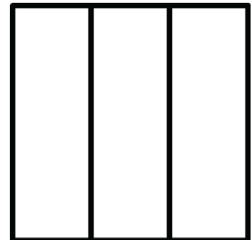
Color \frac{1}{3}
