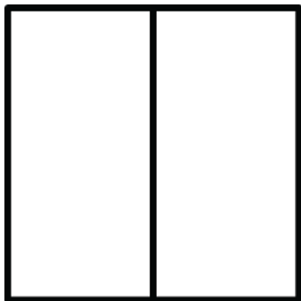
Color \frac{2}{2}
