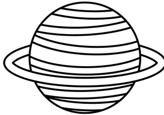
URANUS
