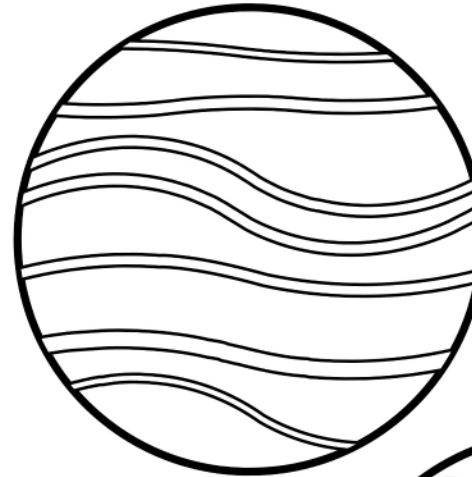
JUPITER
