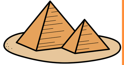
pyramid
