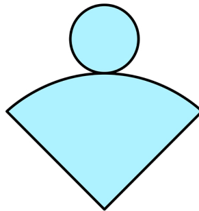
cone
