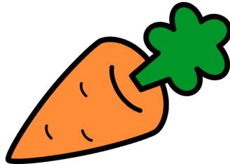
cone
